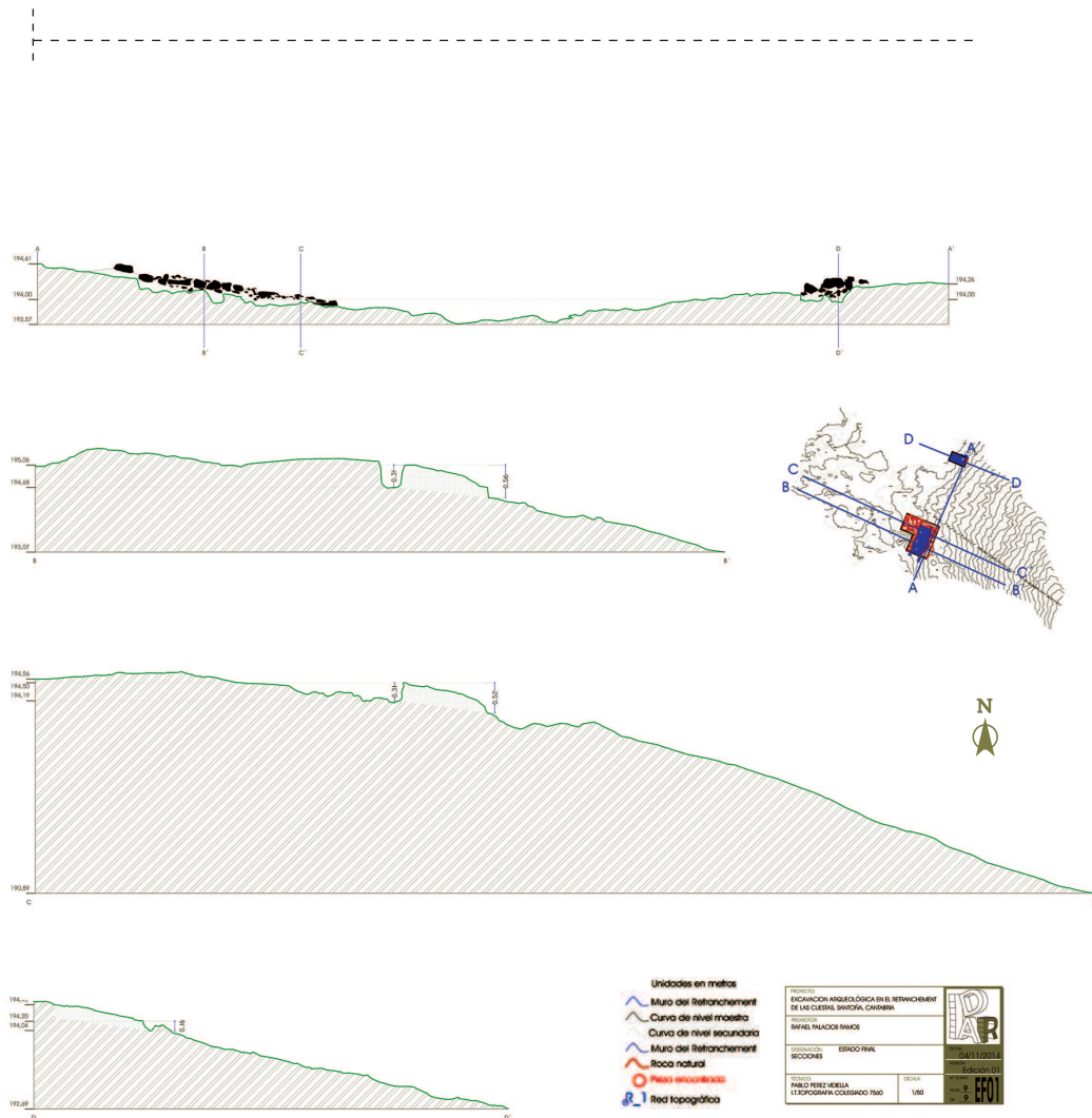
Figura 8. Secciones longitudinales y transversales del terreno y parapeto (escala 1:20).
